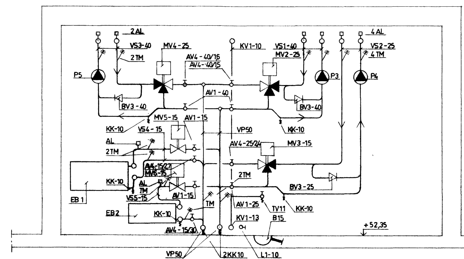
B-B SKALA 1:20
